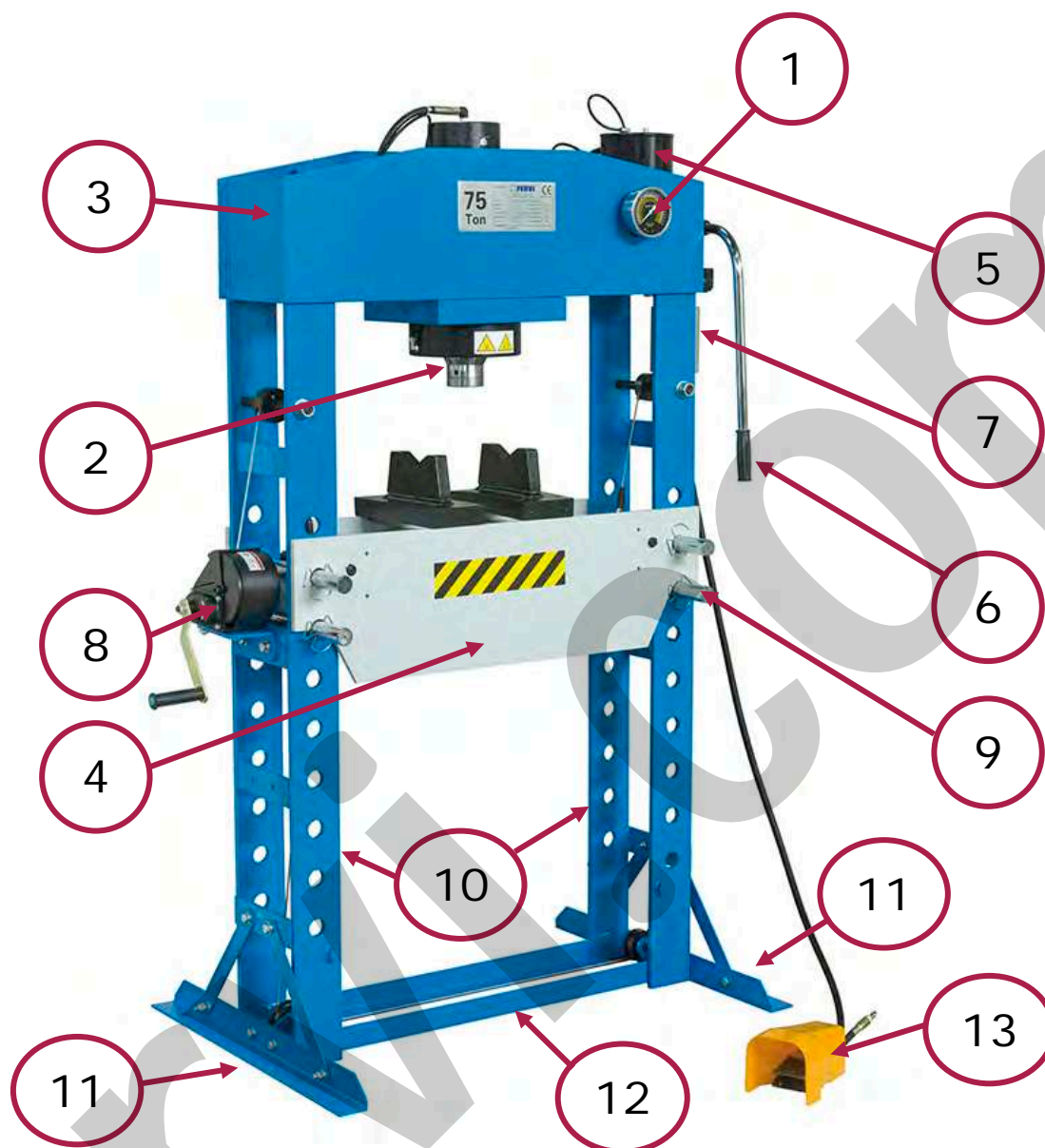
Figura 1 - Vista generale
